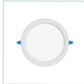
EB-9376 (22W) Size : Ø220x48mm Cut-Out : Ø205mm
